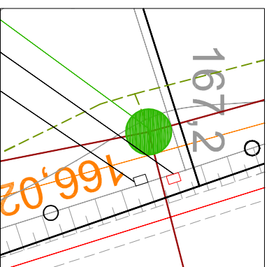
Przepompownia PS3 dz. nr 32/1 skala 1:250 SZCZEGÓŁ A
